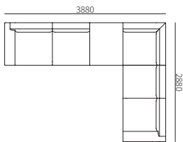
L186ZH-7 3880*2880*720mm 152.8*113.4*28.3"
