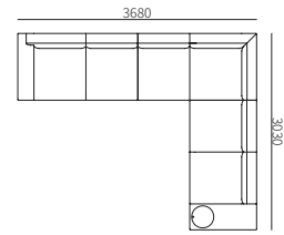
L186ZH-6 3680*3030*720mm 144.9*119.3*28.3"
