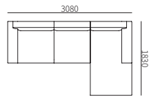
L186ZH-2 3080*1830*720mm 121.3*72.0*28.3"
