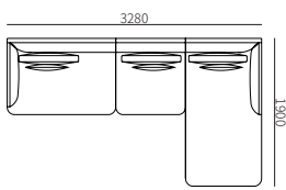
YH25ZH-4 3280*1900*745mm 129.1*74.8*29.3"
